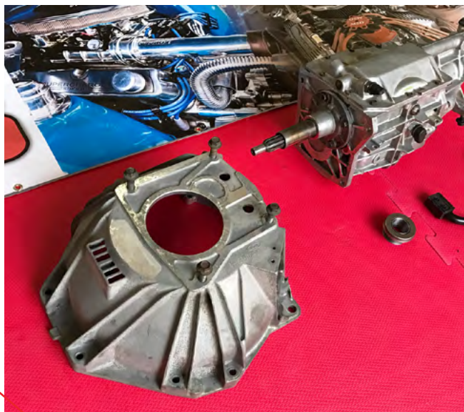
Câmbio Tremec T5 Ford Maverick
